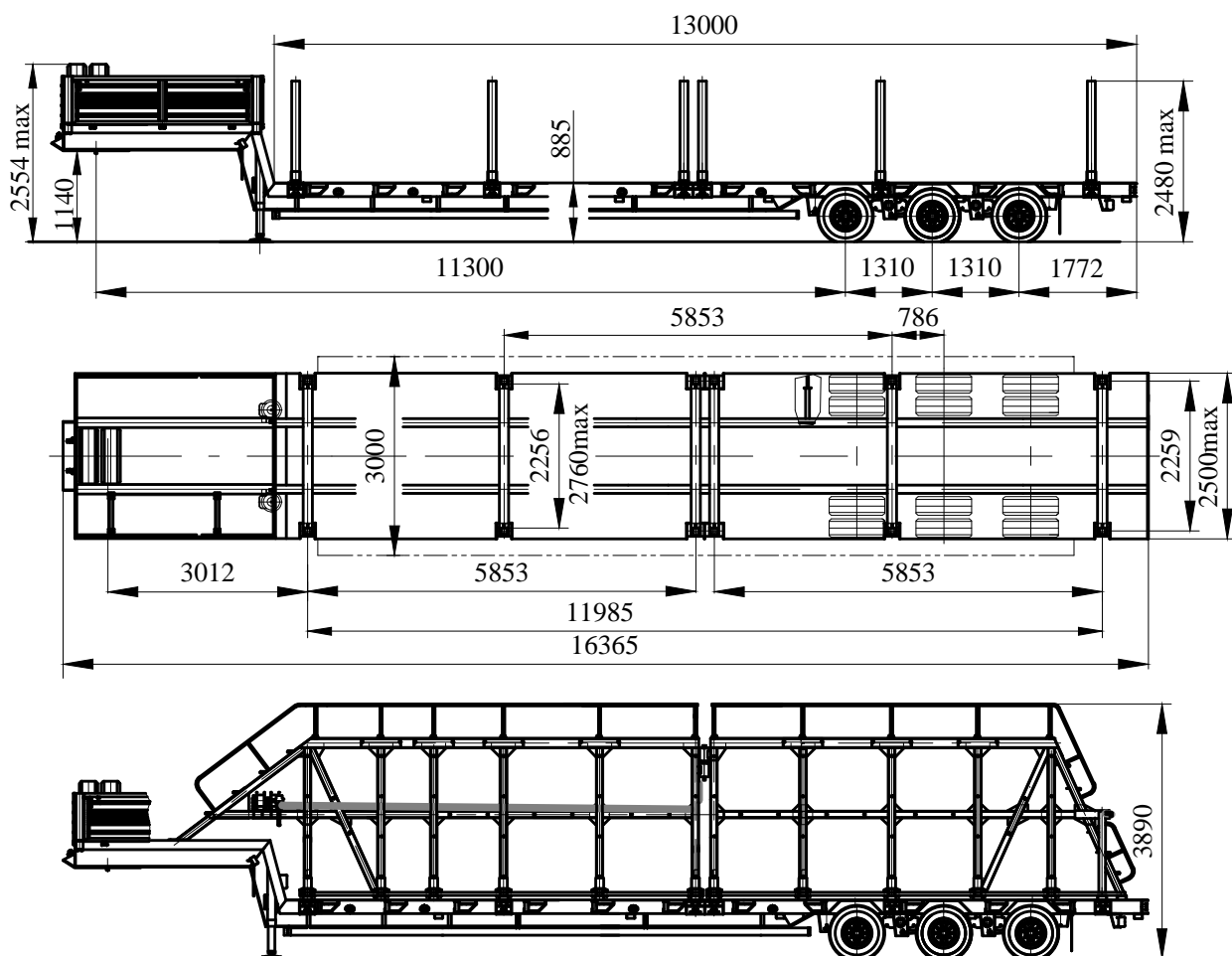
Размеры при полной массе полуприцепа
